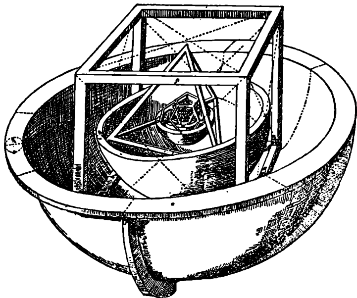
Modelo Keplero de los sólidos regulares
