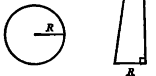
Relación de Arquímedes entre el círculo y el triángulo
